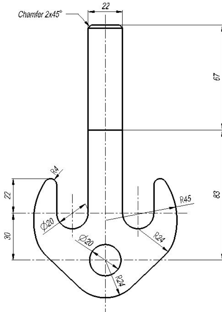
Prob.3-13. Hook
