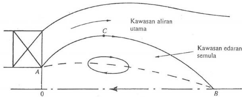
Rajah1 Kawasan Edaran Semula Dalam Medan Aliran Pusar [2]
