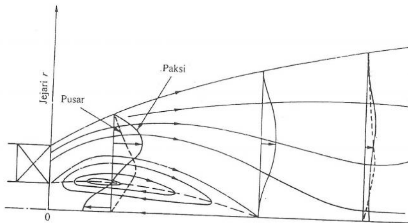
Rajah 2 Susuk Biasa Komponen Halaju Paksi dan Pusat Dalam Medan Aliran Pusaran yang Kuat [2]
