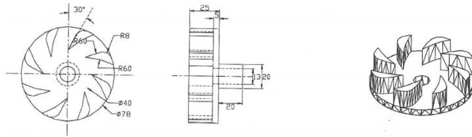
Pemisar Udara 30°
