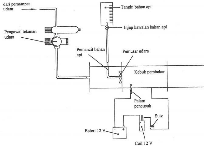
Rajah 6 Rig Ujikaji Pembakar Jenis Kaleng
