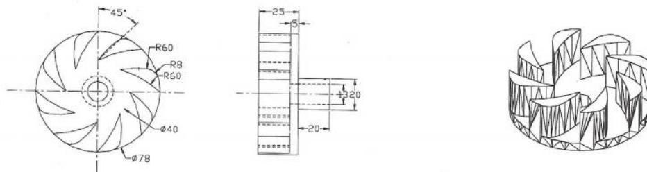
Pemisar Udara 45°
